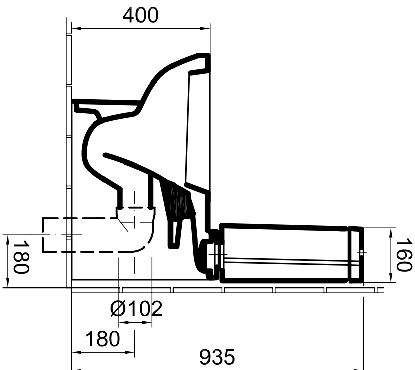
8767 00 00 Átlatkító könyökcső
